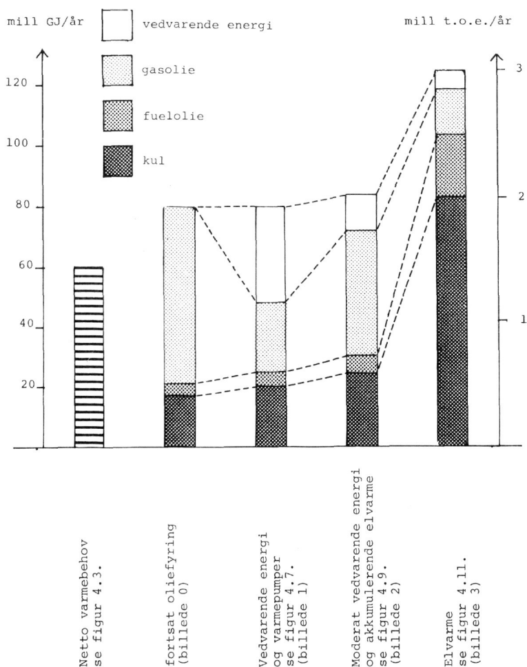
Figur 10.5 Område IV's nettovarmebehov og de tilhørende brændselsforbrug i 1995 i de 4 fremtidsbilleder.
