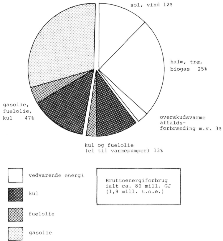
Figur 10.2 Område IV's brændselsforsyning i 1995 ved kraftig udbygning med vedvarende energi og varmepumper (billede nr. 1).
